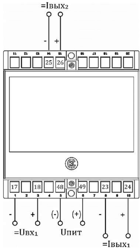
б) Корпус E20 (1 вход, 2 аналоговых выхода)
