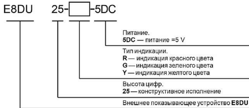
Рисунок 2 – Схема условного обозначения E8DU
