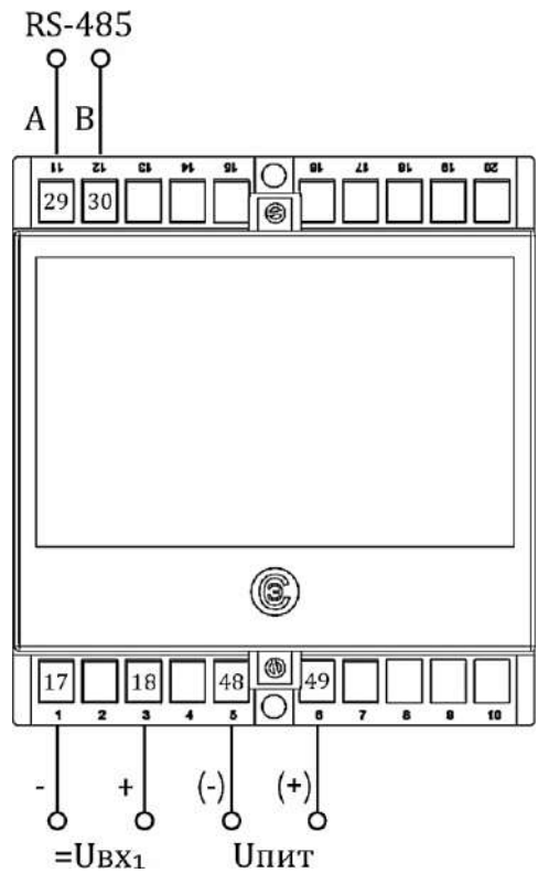
б) Копус E20 (1 вход, 1 порт RS-485)
