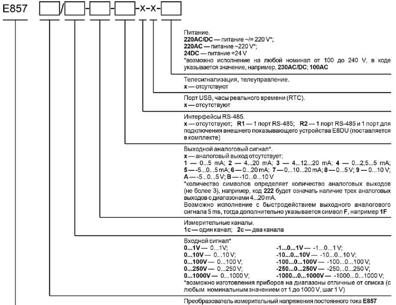
Рисунок 1 – Схема условного обозначения ИП (подробное описание корпусов и возможных исполнений указано в п. 2.16)
